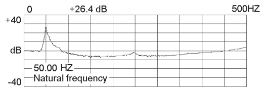
固有振動数
